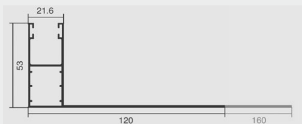
1484 Pala 120mm.
